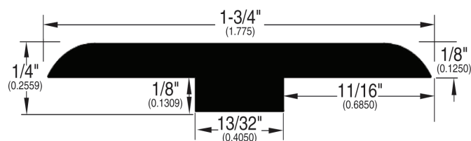
T-Mold (299)
